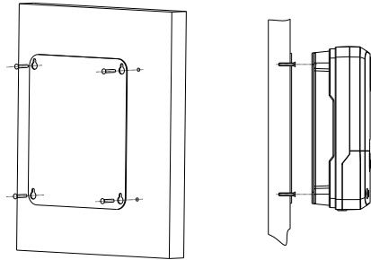
图2.2 固定控制器
