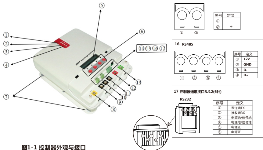
图1-1 控制器外观与接口
