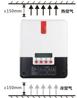
图2.1 安装和散热
