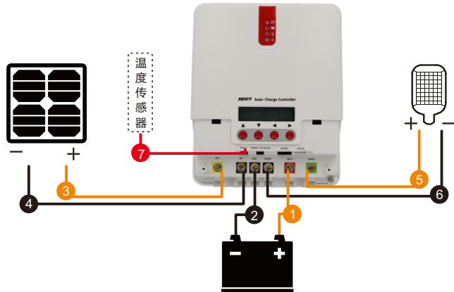
图2.3 接线顺序
