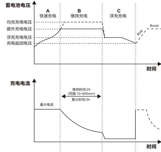
图1-5 蓄电池充电阶段示意图
